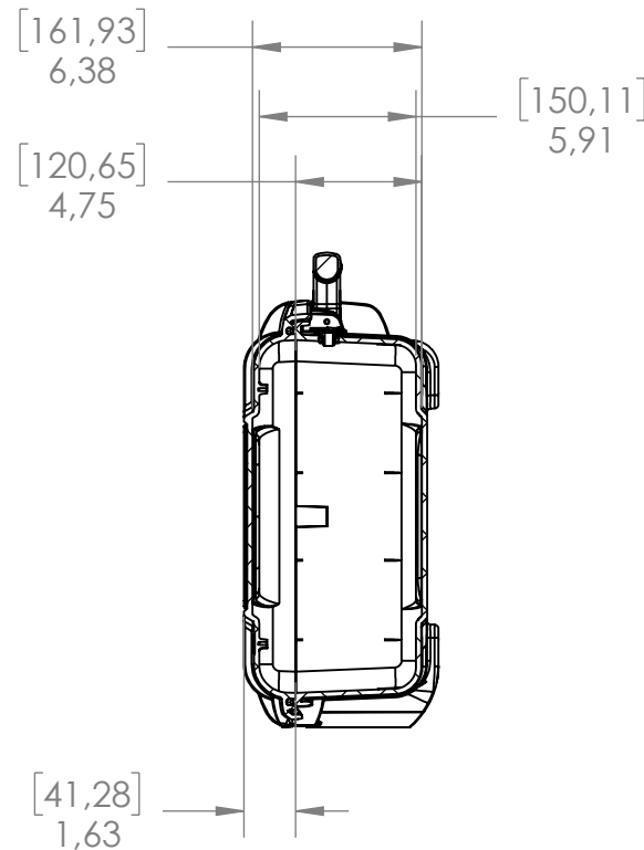
SECTION B-B SCALE 1 : 8
